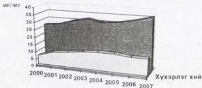
□ Хүхэрлэг хий ■ Азотын давхар исэл
